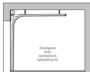
Prowadzenie Standardowe Podwyższone NH (sprężyny skrętne z przodu)
