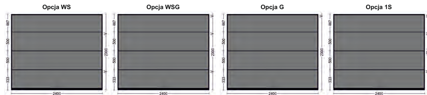
Bramy E130 – wykonanie opcjonalne (wym. spec.) Bramy ze sprężynami skrętnymi - standardowe wykonanie - panel ścięty symetrycznie do dolnego i okuty profilem aluminiowym
