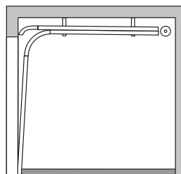
Prowadzenie Obniżone L (sprężyny skrętne z tyłu)
