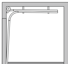
Prowadzenie Standardowe N (sprężyny skrętne z przodu)
