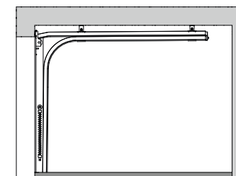
Prowadzenie E130 (sprężyny naciągowe)
