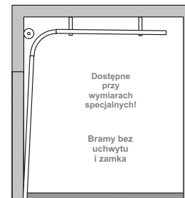
Prowadzenie Wysokie H (sprężyny skrętne z przodu)
