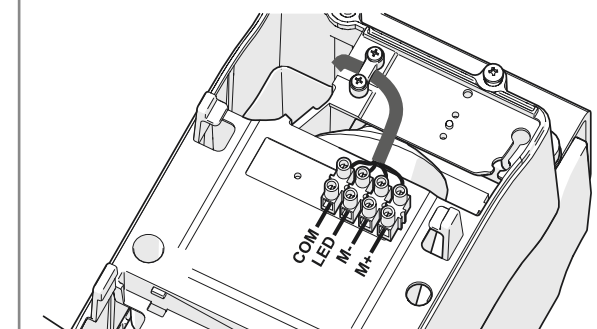
Połączenia elektryczne - ARTO PRO
