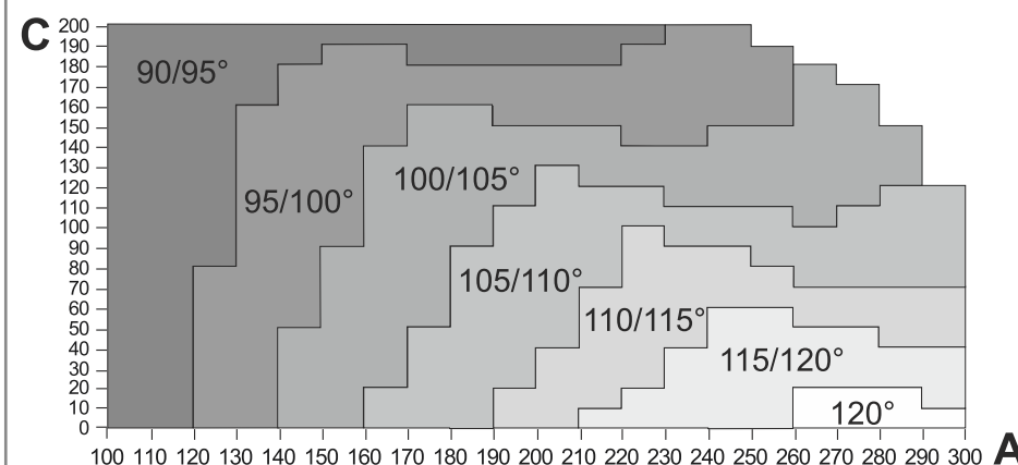
Wykres kąta otwarcia
