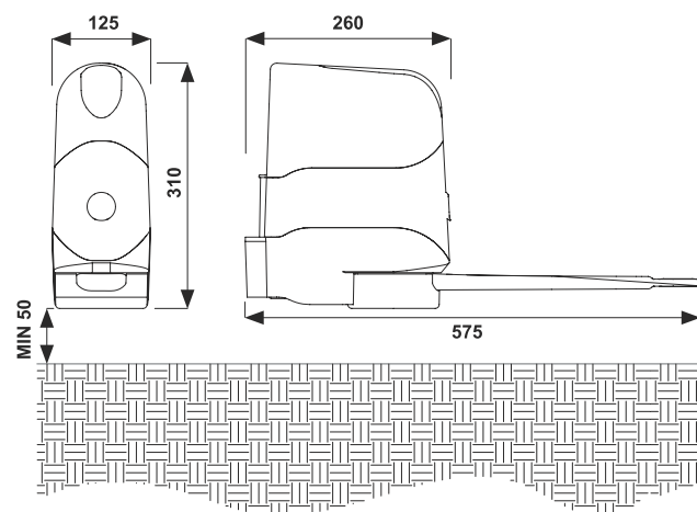
Wymiary
