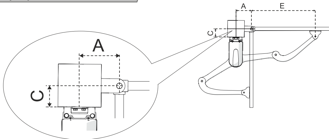
Wymiary montażowe
