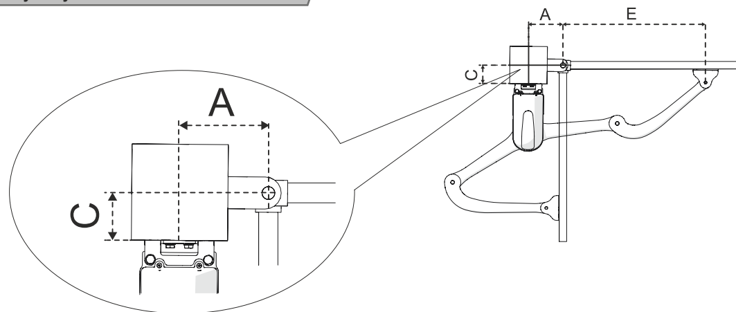
Wymiary montażowe
